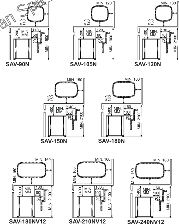
Abb. 2 Fig. 2 Minimale Sicherheitsabstände Minimum Safety Distances
