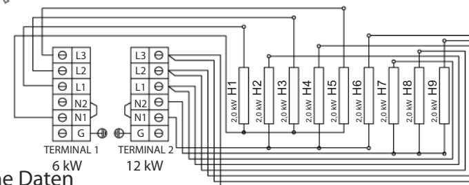
Abb.5 Technische Daten Fig.5 Technical Data
